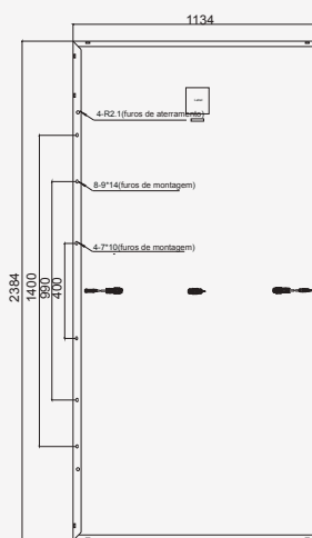
Vista Traseira
