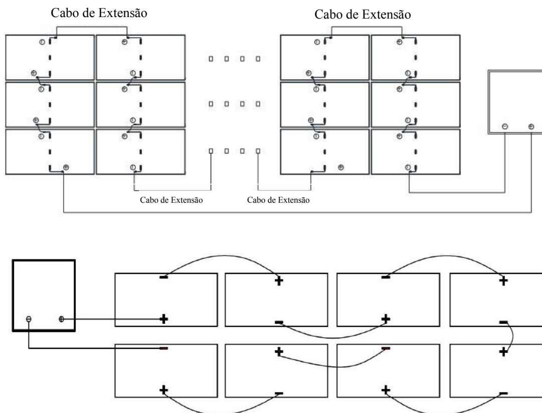
Fig. 5-5 Divisão da J-Box na posição intermediária do módulo para direção horizontal
