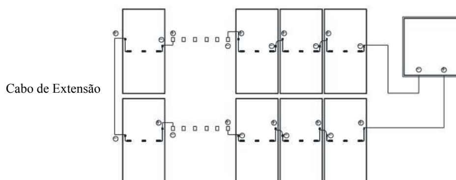
Fig. 5-4 Split J-Box na posição intermediária do módulo para direção vertical
