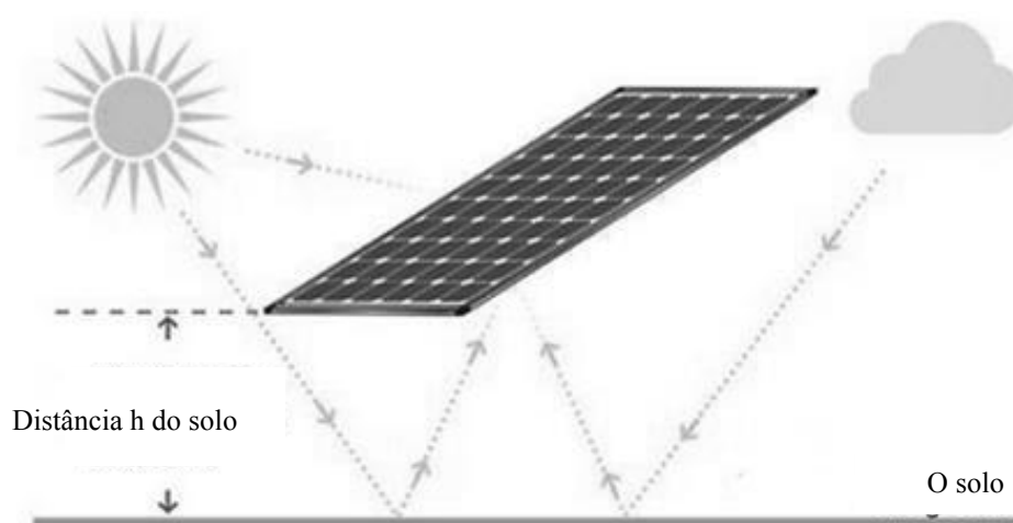
Fig. 5-2 Distância da Terra
